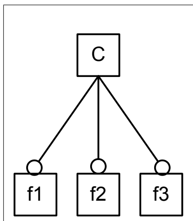
Abbildung 2.4: Variationspunkt: Optionale Feature [CEC00]
