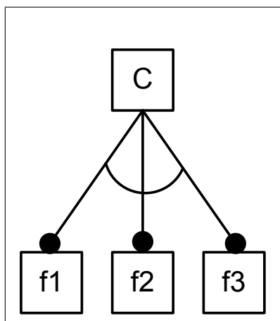
Abbildung 2.5: Variationspunkt: Alternative (obligatorisch) [CEC00]
