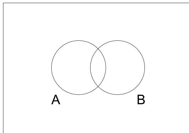
Abbildung 3.9: Optional-Featureproblem[Käs07]
